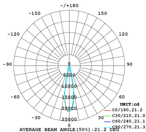
Medium (21°) at 39W
