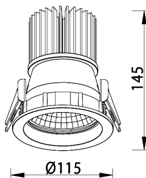
30W/37W Dimensions
