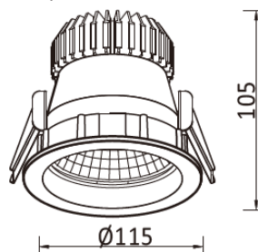
30W/37W Dimensions
